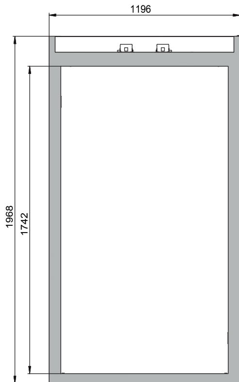
Vooraanzicht
